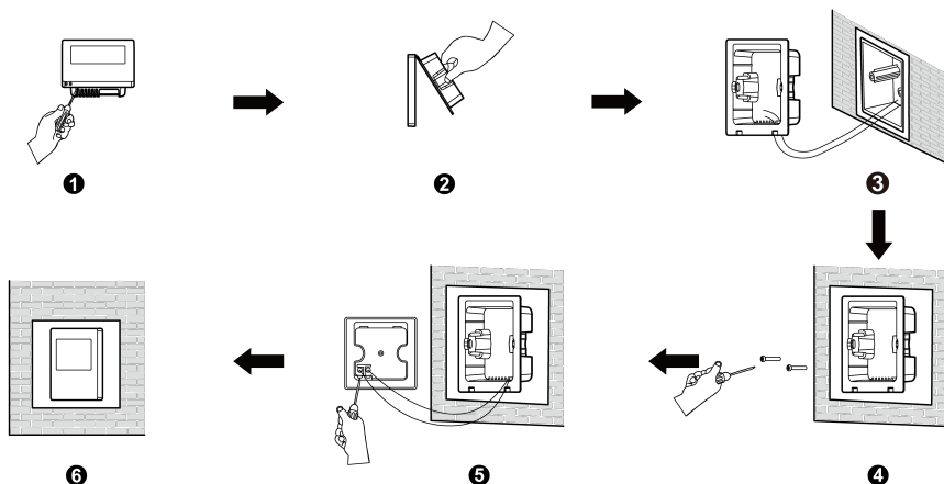
Рис. 7-3 Монтаж дротового контролера
