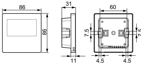
Рис 7-1 Розміри дротового контролера
