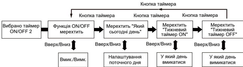
Рис. 5-9 Налаштування кроків тижневого таймера
