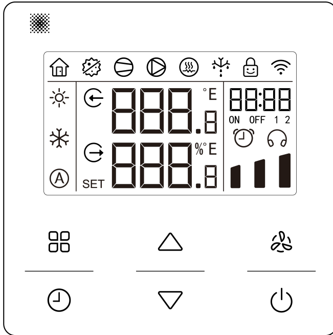
Рис. 2-1 Зовнішній вигляд дротового контролера
