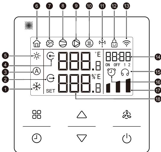
Рис. 2-2 РК-дисплей дротового контролера Таблиця 2.2.1 Опис РК-дисплея
