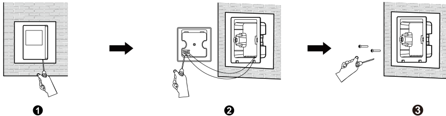
Рис. 7-4 Зняття дротового контролера
