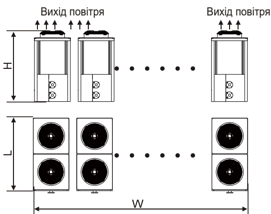
Розміри блоку
